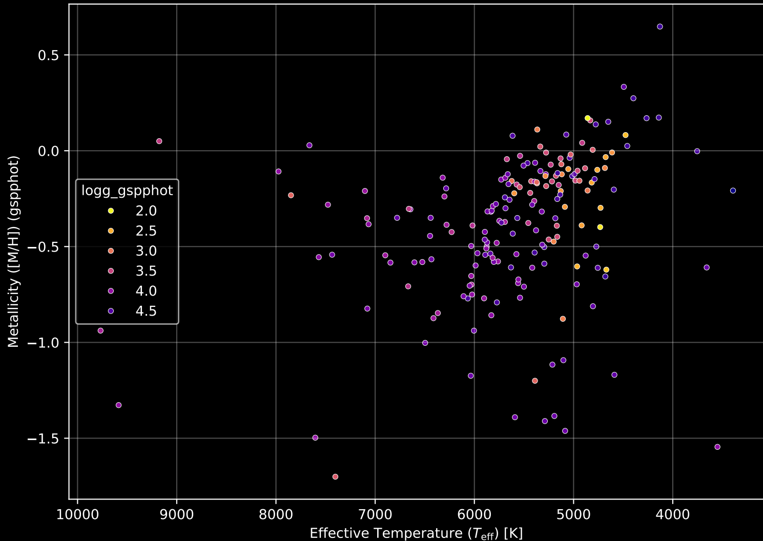
APOGEE DR17 Field: [K2_C13_180-15_btx] Stellar Population Parameters (n= 187)
